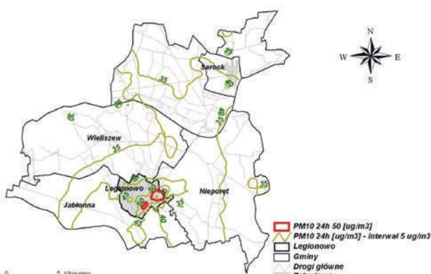
Rysunek 3.57 Rozkład stężeń pyłu zawieszony PM 10 o okresie uśredniania wyników pomiarów 24 godzinny, powodowanych emisją całkowitą, w powiecie legionowskim w 2006 roku
